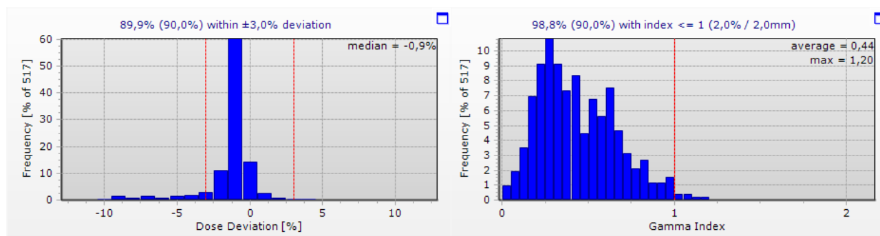
Risultati senza monitoraggio della temperatura (la differenza di temperatura è di 3 °C)
